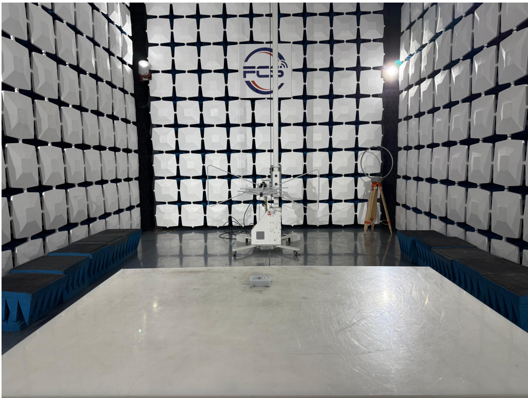
RE (Below1GHz)
