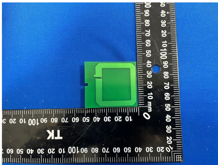
NFC Antenna
