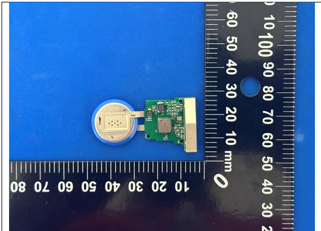
Antenna
