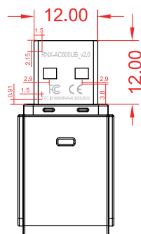
结构图
