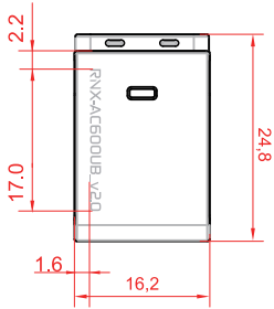
尺寸图
