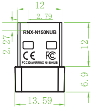
尺寸图
