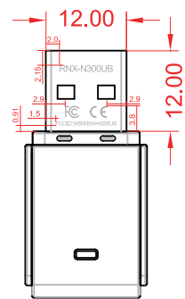
结构图
