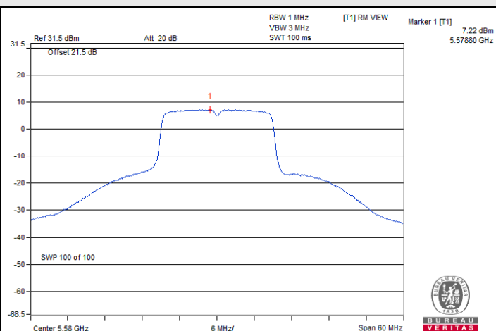
802.11n (HT20) : CH 116
