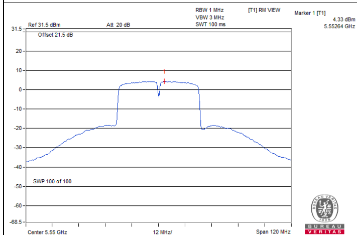
802.11n (HT40) : CH 110
