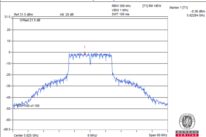
802.11a : CH 165
