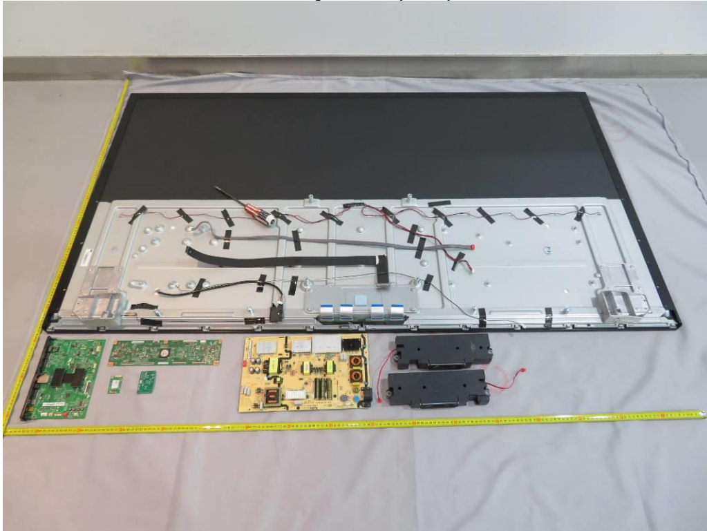
T750QVR04.0 (AUO)
