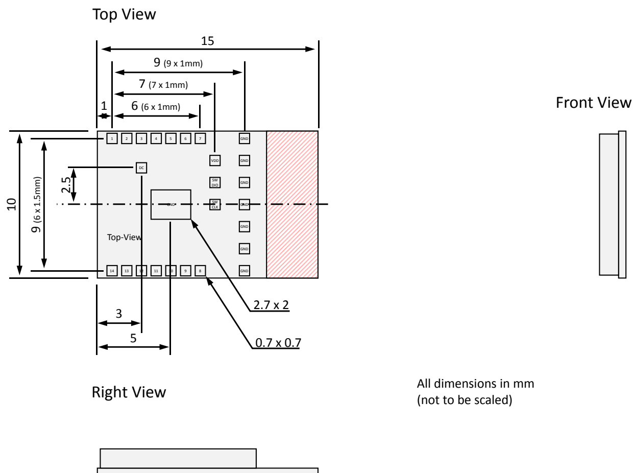
Image 3 Module dimensions
