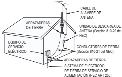
EJEMPLO DE ANTENA A TIERRA SEGÚN EL CÓDIGO ELÉCTRICO NACIONAL, ANSI / NFPA 70
