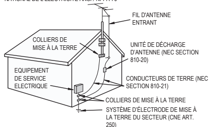
NEC — CODE NATIONAL DE L'ÉLECTRICITÉ
