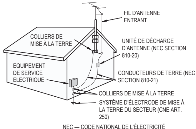
EXEMPLE DE TERRE ANTENNE SELON LE CODE NATIONAL DE L'ÉLECTRICITÉ ANSI / NFPA 70
