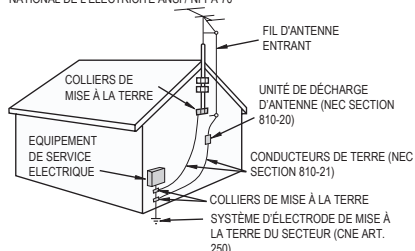
EXEMPLE DE TERRE ANTENNE SELON LE CODE NATIONAL DE L'ÉLECTRICITÉ ANSI / NFPA 70
