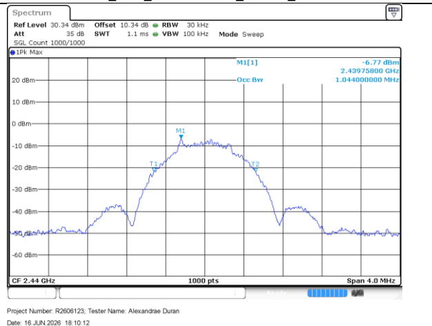
BLE 1M 2440MHz OBW 99%
