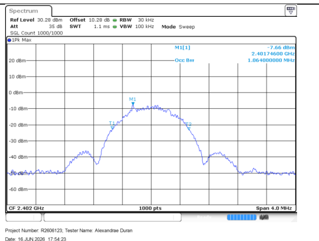
BLE_1M_2402MHz_OBW_99%
