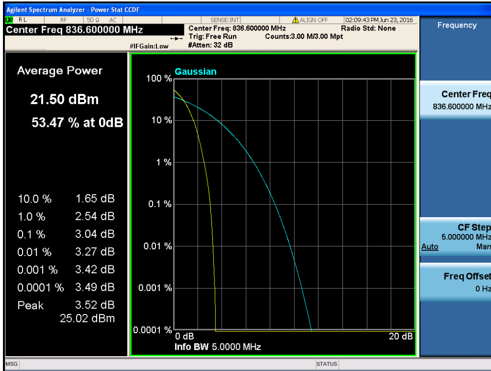
WCDMA850 & Channel: 4183
