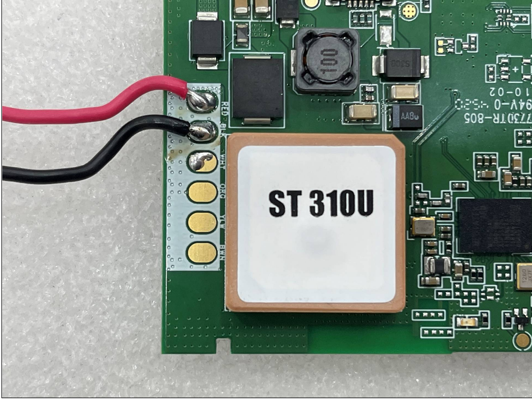
GPS Module
