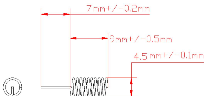
尺寸图
