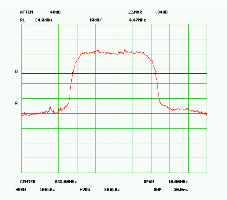
W850-26dB-M
