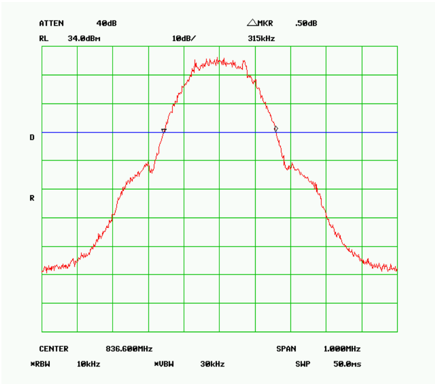
850-26dB-M
