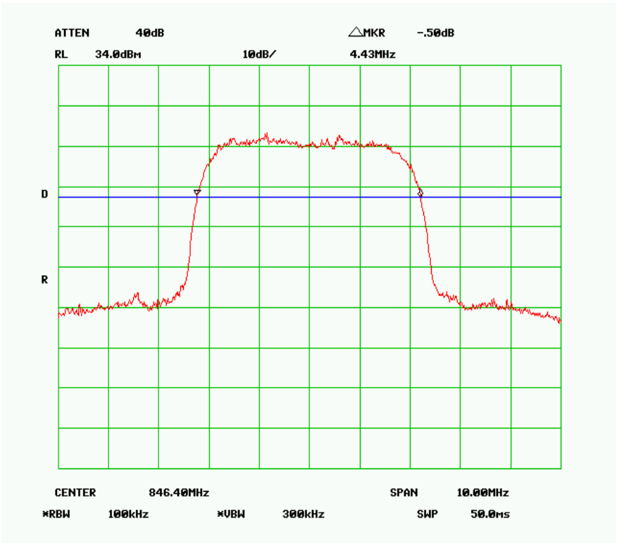
W850-26dB-H
