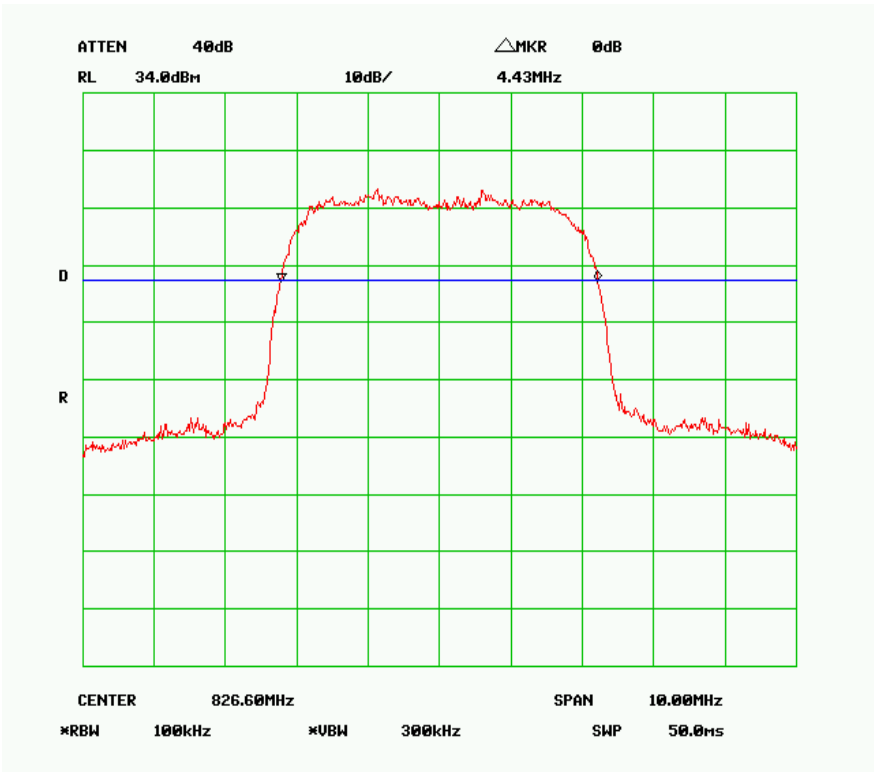
W850-26dB-L
