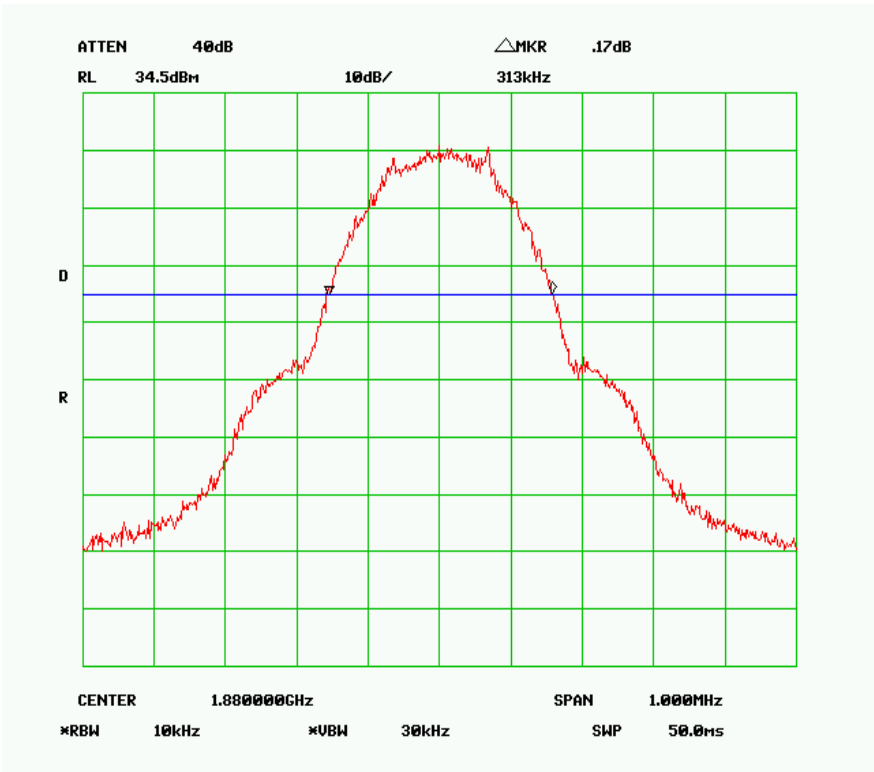
1900-26dB-M
