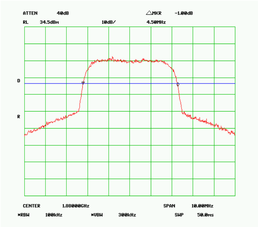
W1900-26dB-M
