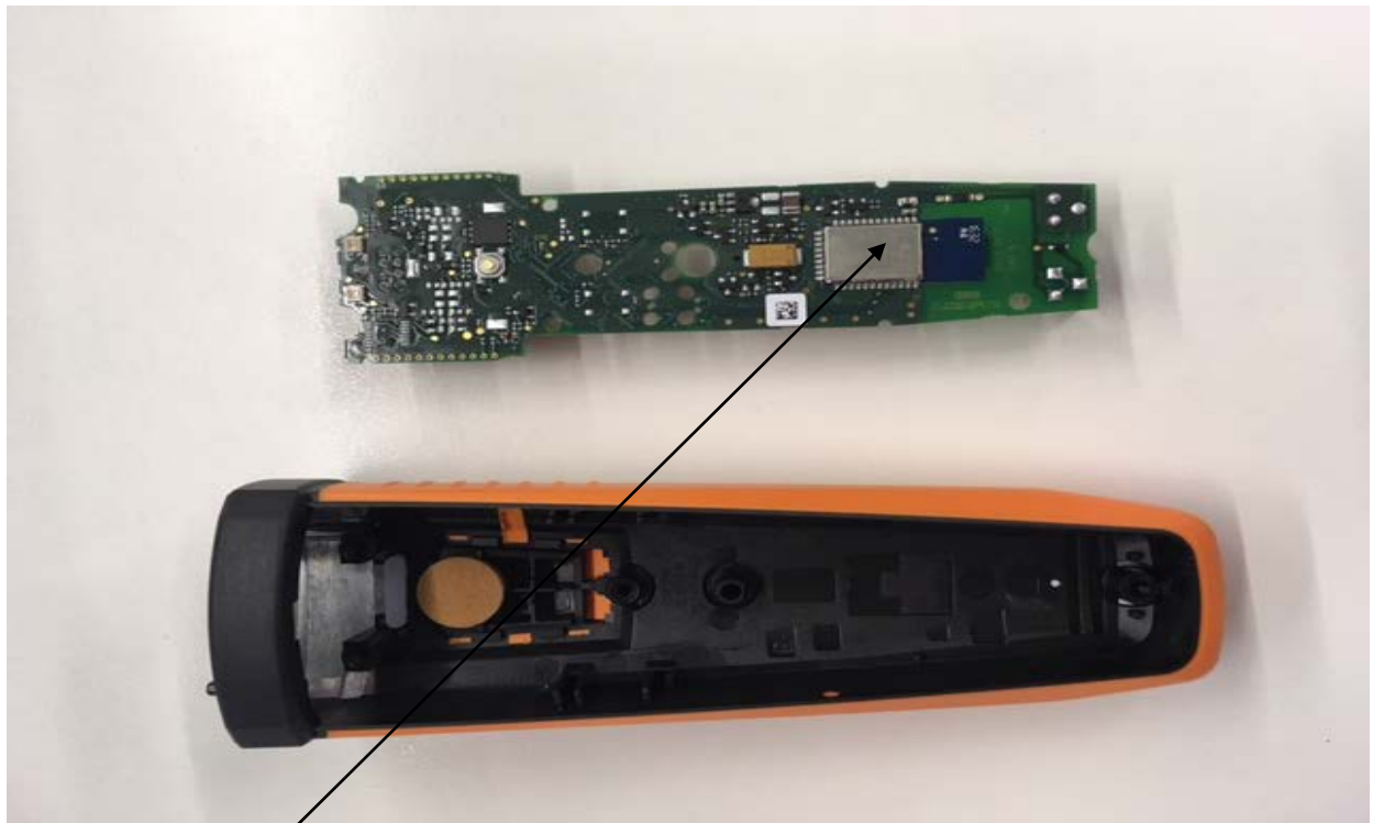
Module + Antenna
