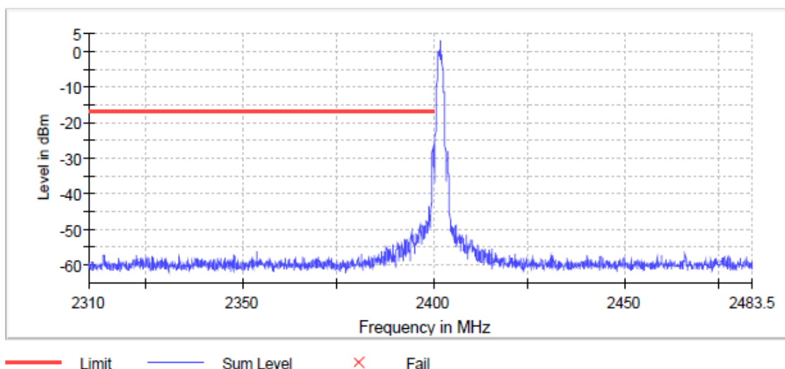
BT LE 2 Mbps Ch 00 Band Edge
