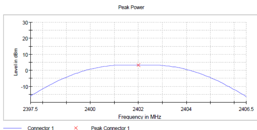
BT LE 2 Mbps Ch 00
