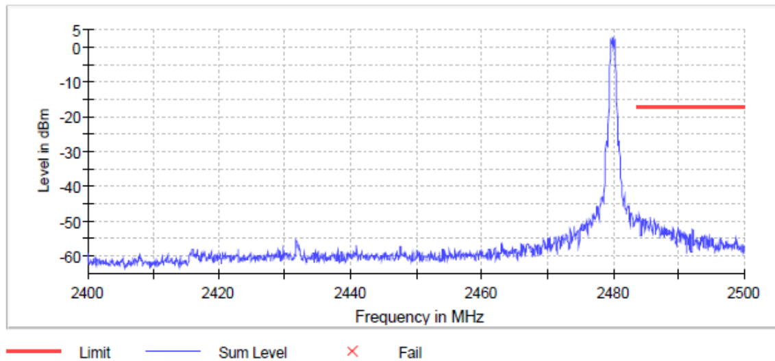
BT LE 1 Mbps Ch 39 Band Edge
