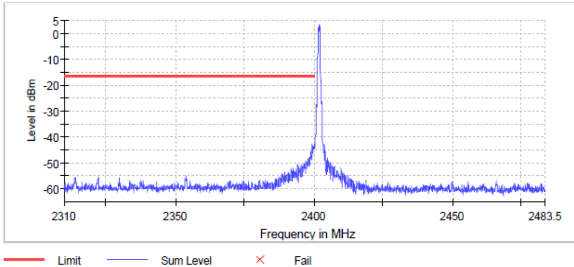
BT LE 1 Mbps Ch 00 Band Edge
