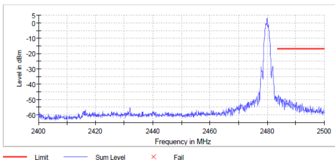
BT LE 2 Mbps Ch 39 Band Edge
