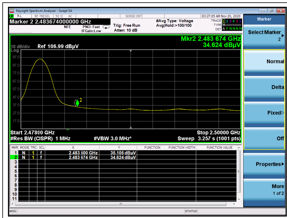
(AVERAGE, Channel 39)
