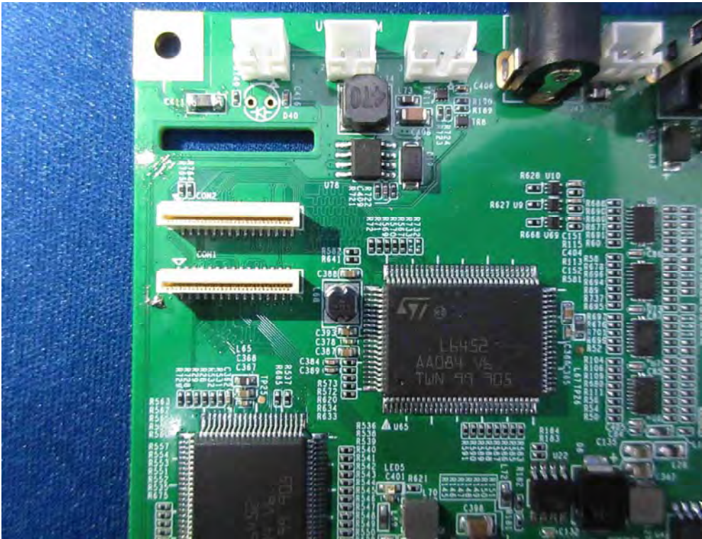
(50) EUT Photo
