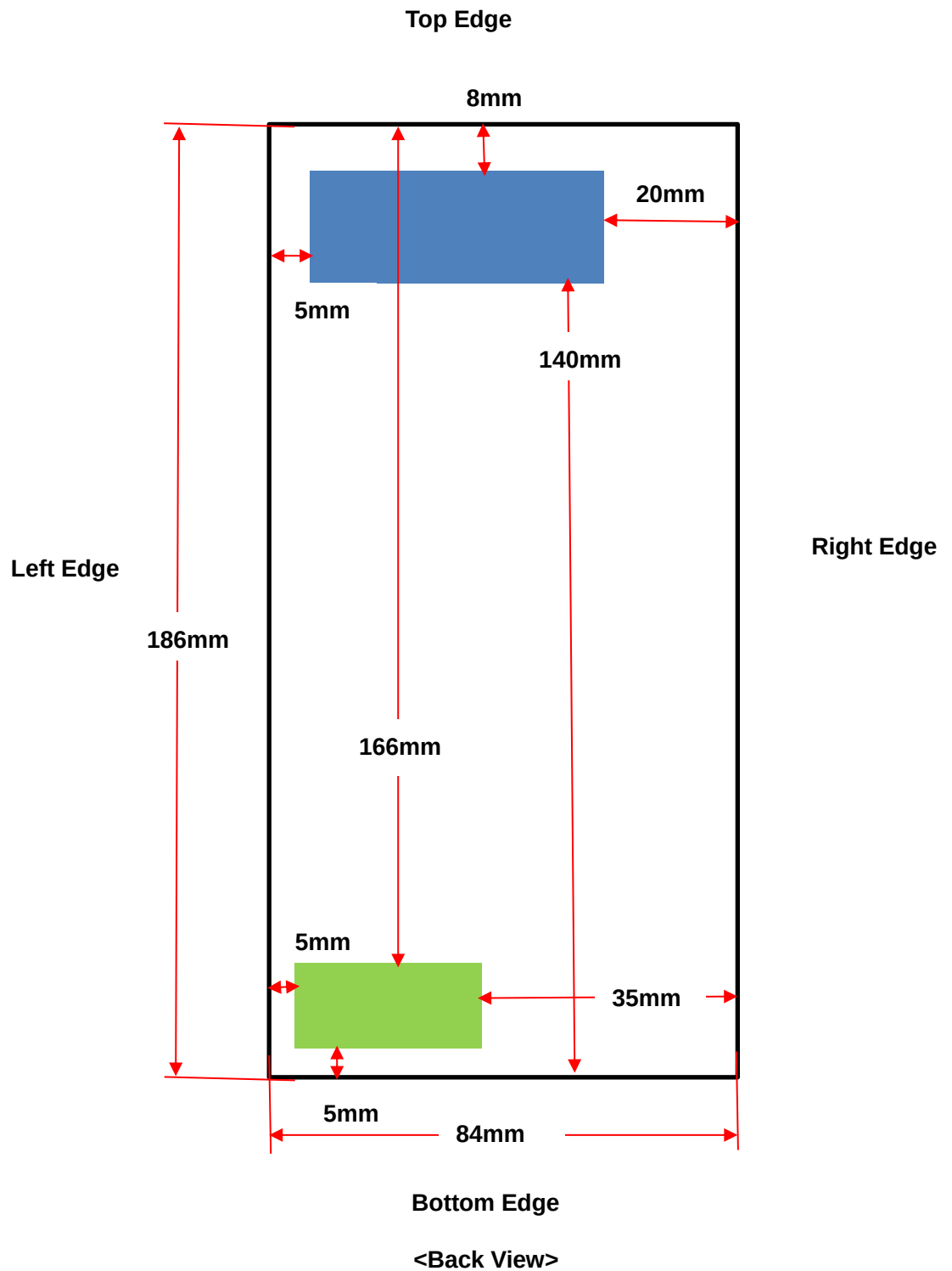
WWAN Antenna
