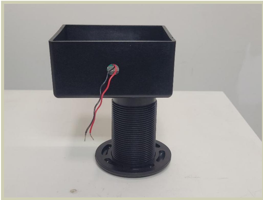
EUT Horizontal
