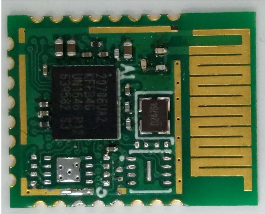
(3) EUT Photo
