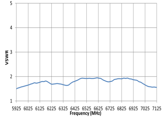
6 / 7 GHz VSWR
