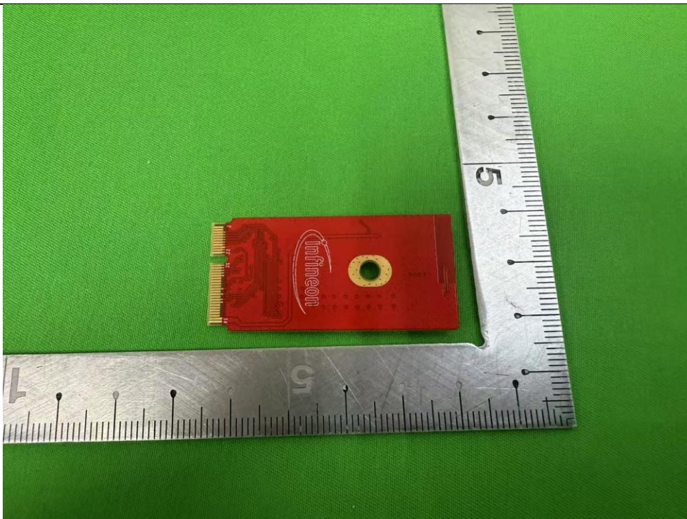
(6) EUT Photo For CYW20829B1-P5CAI100
