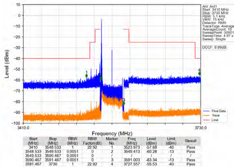
n78d 30kHz MIMO NTV 40MHz CP-OFDM QPSK 3570MHz Edge_1RB Left
