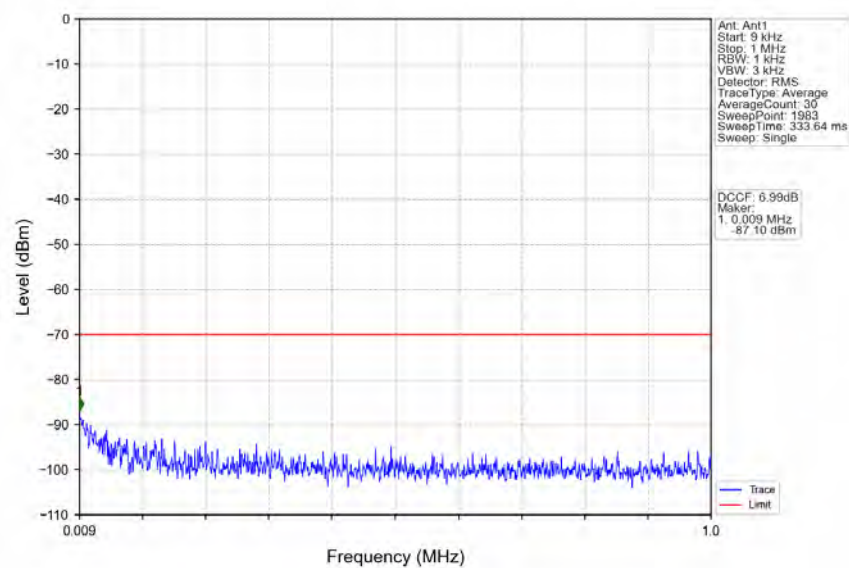
n78d 30kHz MIMO NTV 40MHz CP-OFDM QPSK 3570MHz Edge_1RB Left
