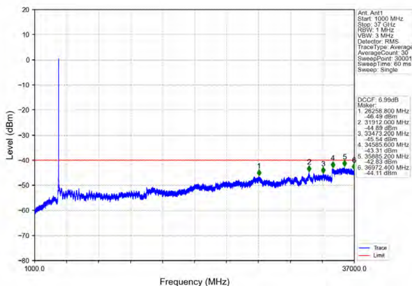
n78d 30kHz MIMO NTNV 20MHz CP-OFDM QPSK 3690MHz Outer Full
