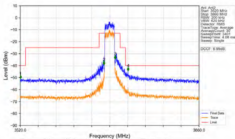
n78d 30kHz MIMO NTNV 20MHz CP-OFDM QPSK 3690MHz Outer Full
