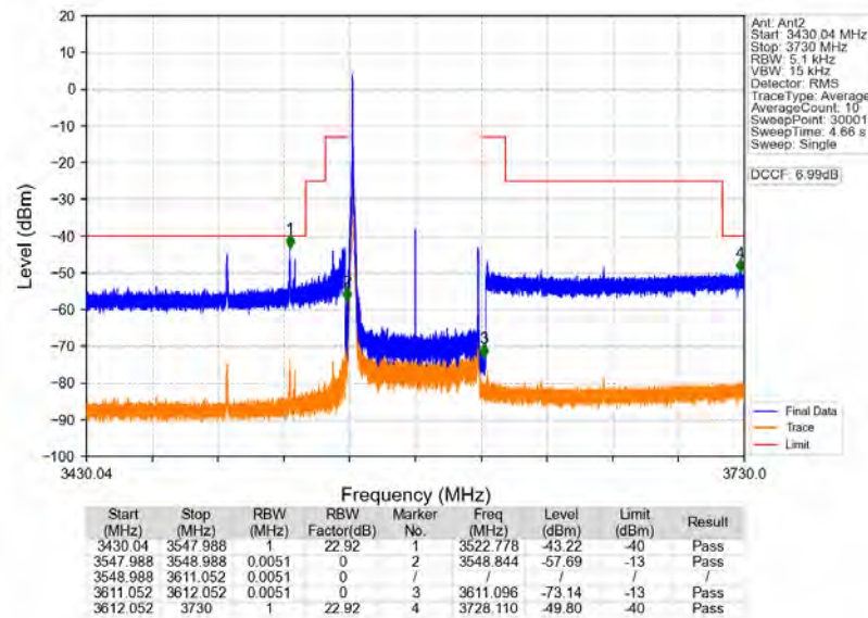
n78d 30kHz MIMO NTNV 60MHz CP-OFDM QPSK 3580.02MHz Inner 1RB Left
