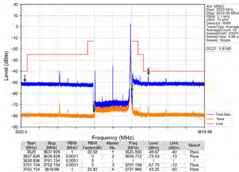
n78d 30kHz MIMO NTNV 60MHz CP-OFDM QPSK 3669.99MHz Edge 1RB Right
