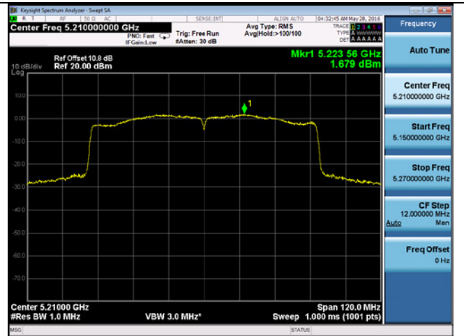
PSD-802.11ac-80M-5210M-chain2
