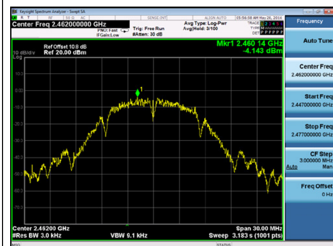
PSD-2.4G-802.11b 2462MHz
