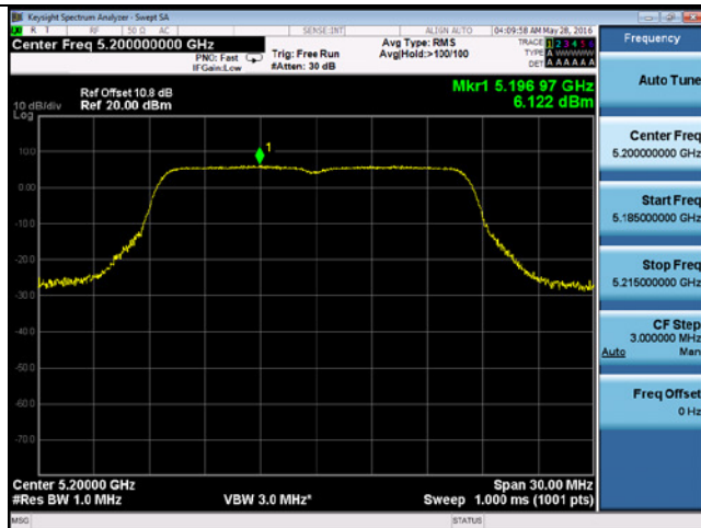
PSD-802.11a-5200M-chain2
