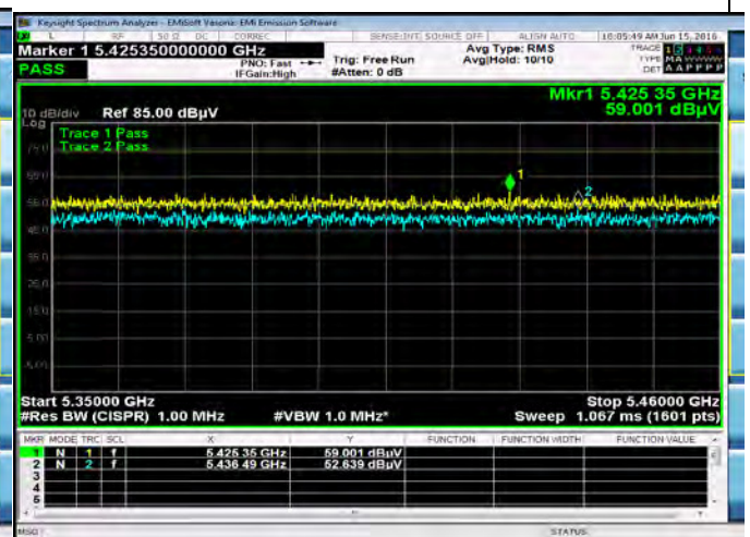
802.11ac 5530M(5350-5460MHz)
