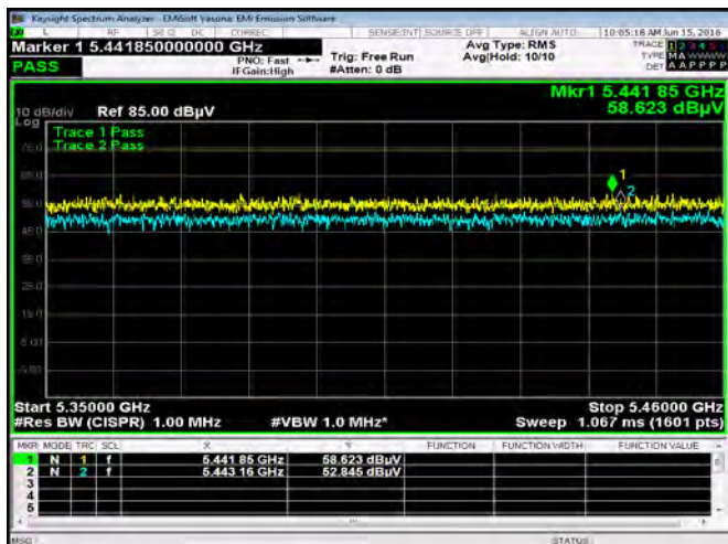
802.11n-HT40 5510M(5350-5460MHz)
