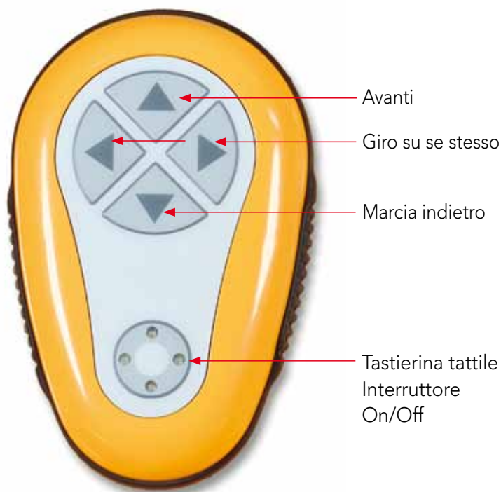
Figura 16: Il Telecomando
