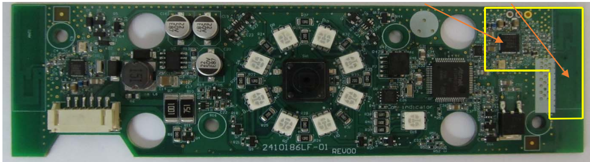
WiFi module. WiFi antenna.
