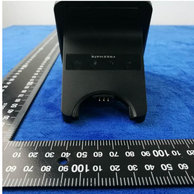
EUT - Top View(FP)
