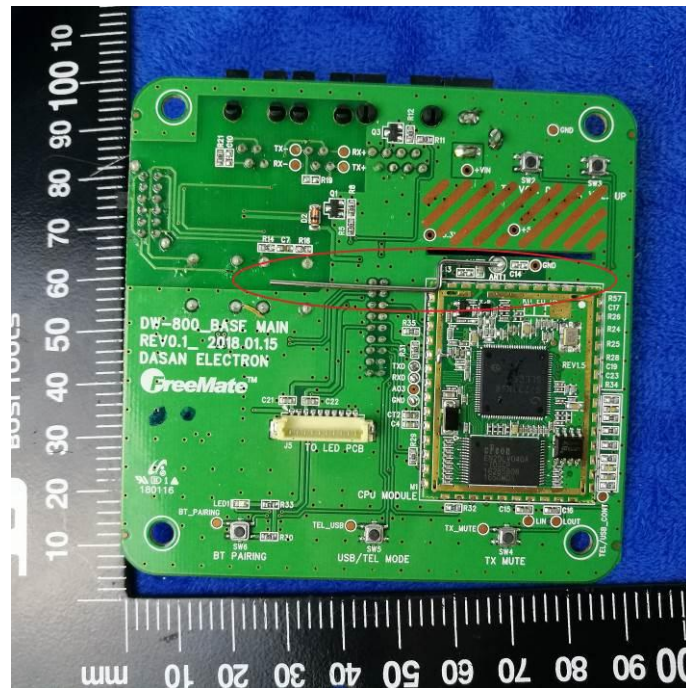
Antenna View(FP)
