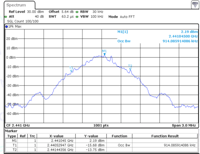
DH5-Ant1-2441
