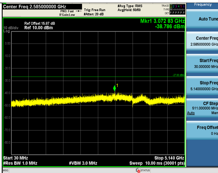
11AC80SISO-Ant1-5210-30~5140-PASS
