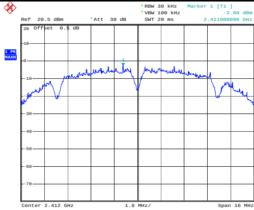
PSD - Low CH 2412-802.11b-(ANT1#)
