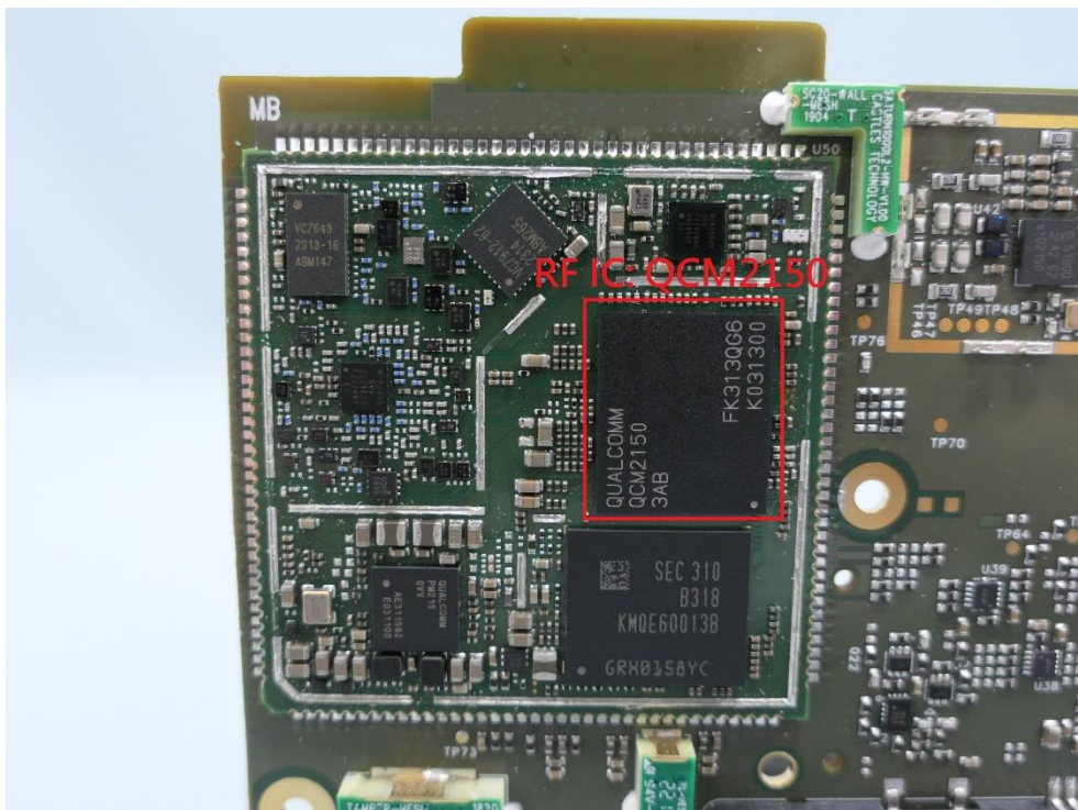
(36) EUT Photo
