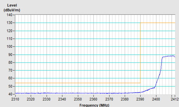
Horizontal (Average)
