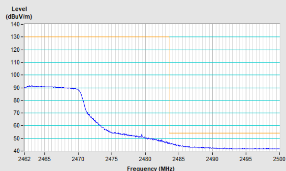
Vertical (Average)
