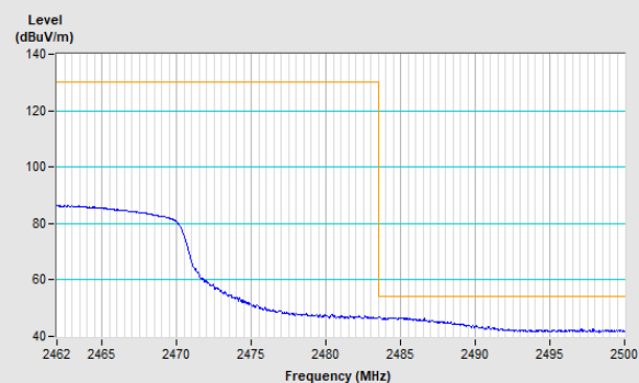
Horizontal (Average)
