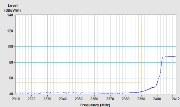
Vertical (Average)
