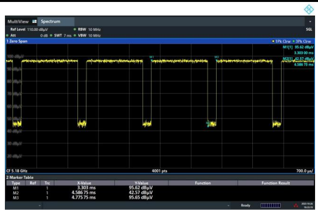
802.11 n20
