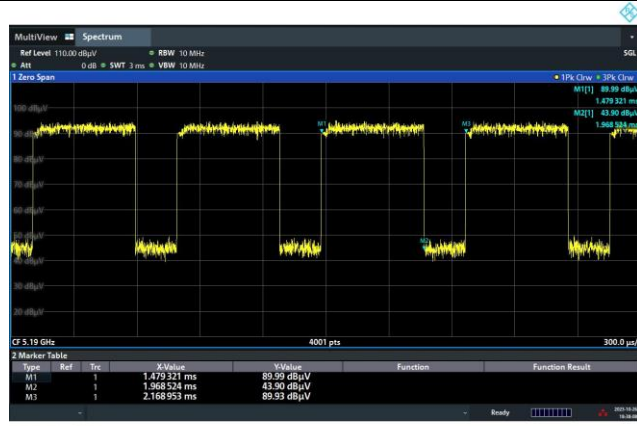
802.11 n40
