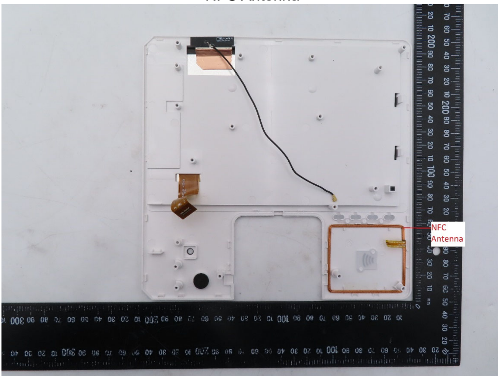
NFC Antenna
