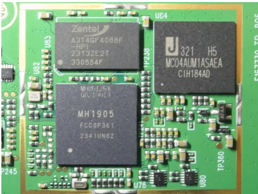
(8) EUT Photo (V1P 3.5)
