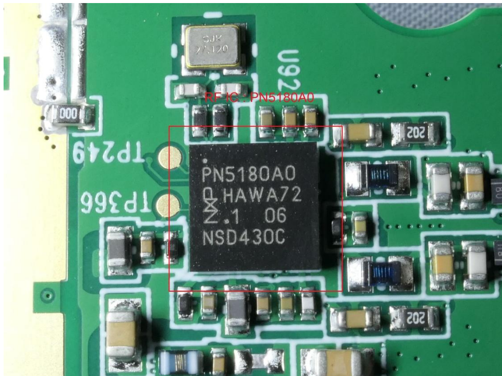
(17) EUT Photo (V1P-BK)
