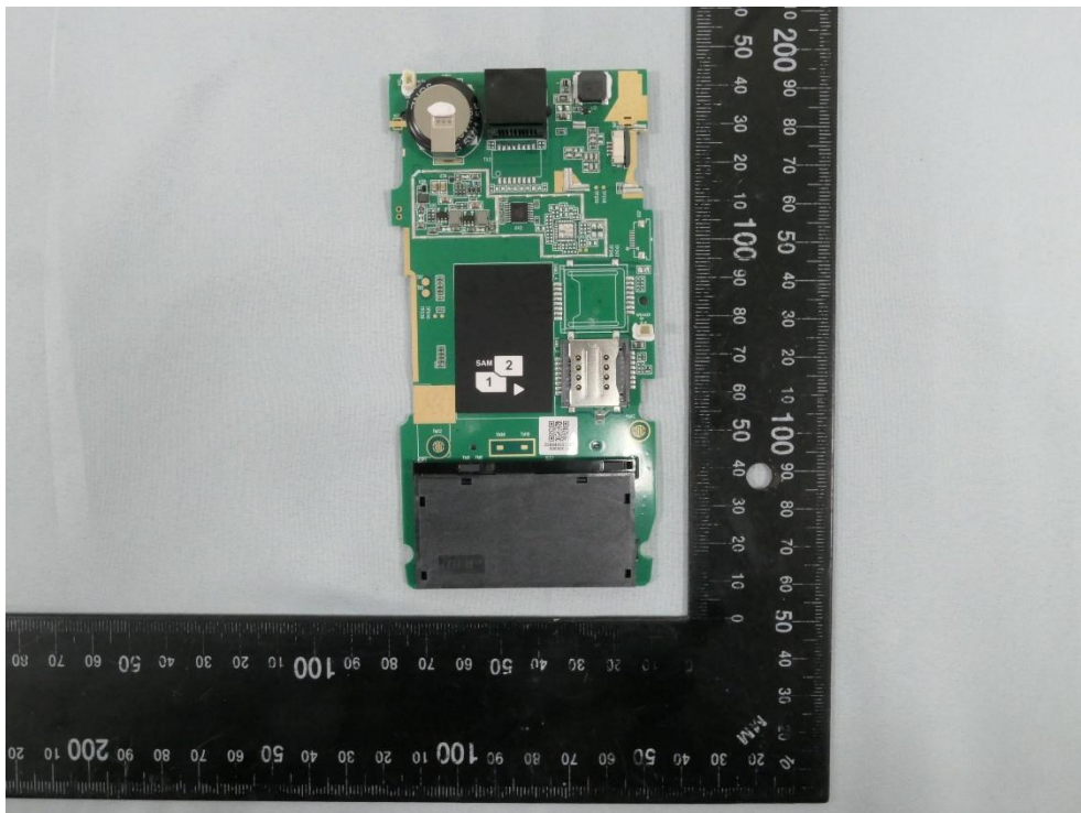
(14) EUT Photo (V1P-BK)
