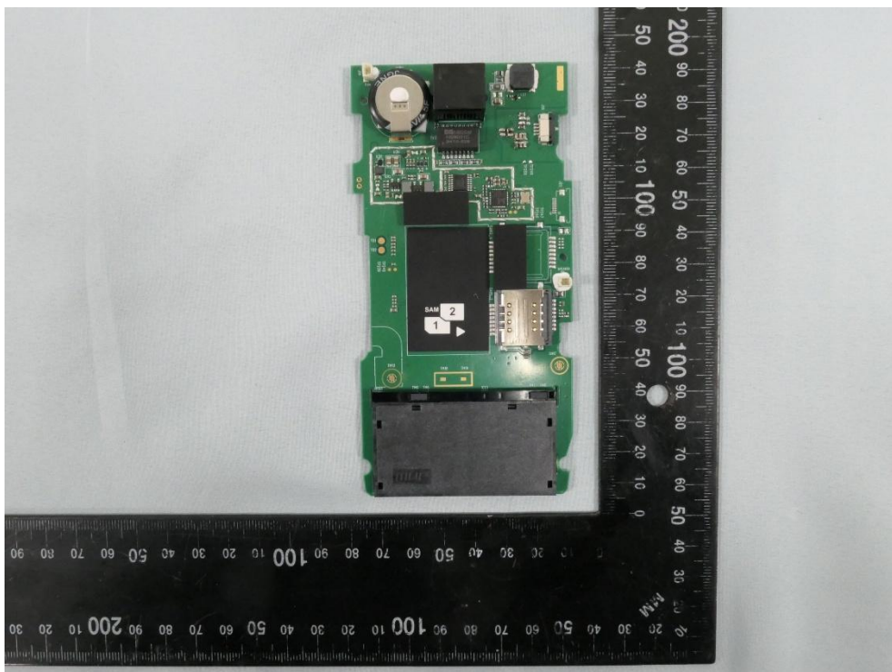
(4) EUT Photo (V1P 3.5)
