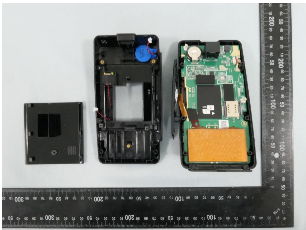
(10) EUT Photo (V1P-BK)
