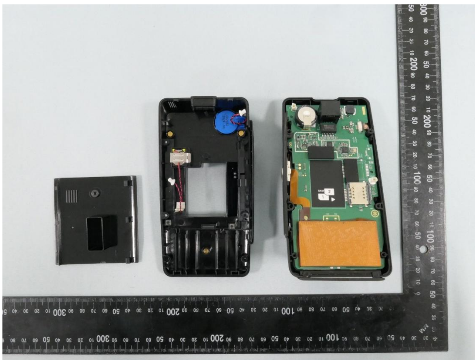
(2) EUT Photo (V1P 3.5)
