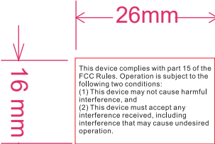
B-TFS00-20 FS警告语贴 亮银龙+哑胶、26*16mm
