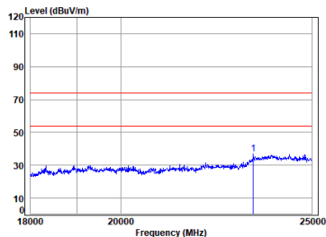
BLE_2M_TX_CH_39_Horizontal
