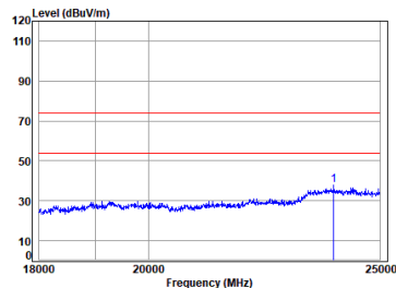
BLE_2M_TX_CH_39_Vertical
