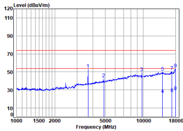
BT_DH5_TX_CH_39_Horizantal
