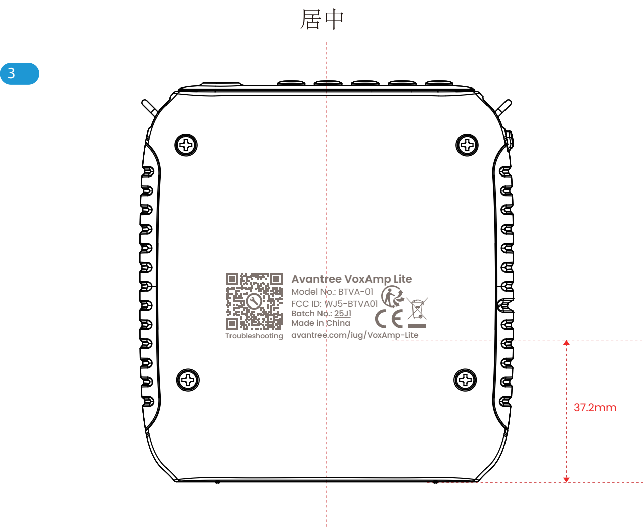
背面丝印
