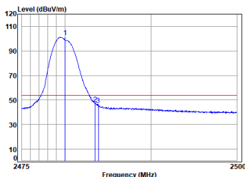
BLE_2M_TX_CH_39_Horizontal-AVG
