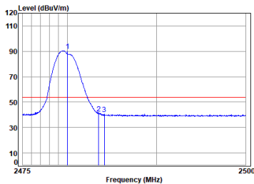
BLE_2M_TX_CH_39_Vertical-AVG
